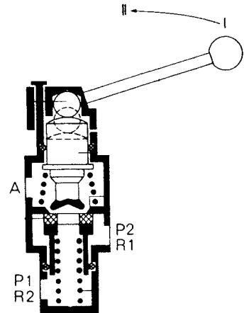
Slika 102. Odzračno-dozračni ventil
