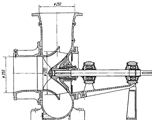
e) presjek jednostupanske dijagonalne sisaljke (8413 70 91 KN-a)
